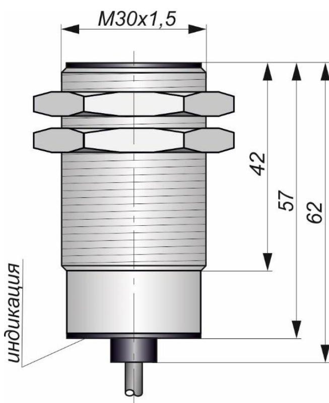
Габаритный чертеж
